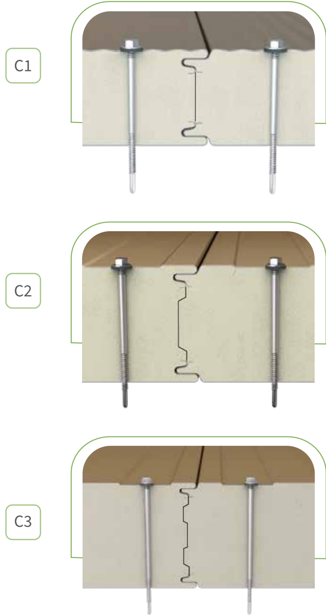
Birleşim Detayı Connection Detail
