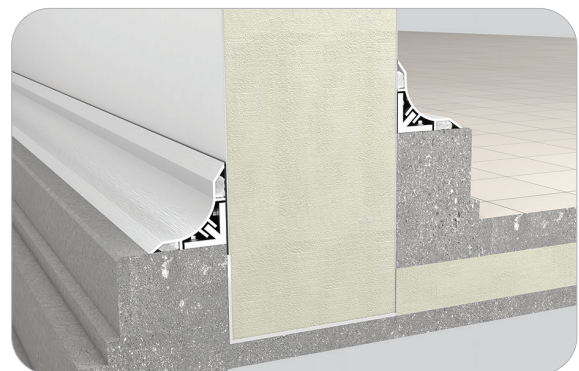
Soğuk Oda Duvar-Zemin Birleşim Detayı / Cold Room Wall-Floor Connection Detail
