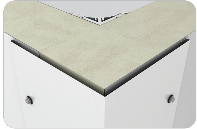
Soğuk Oda Duvar-Zemin Birleşim Detayı / Cold Room Wall-Floor Connection Detail
