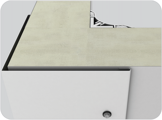
Soğuk Oda İç Köşe Detayı / Cold Room Inner Corner Detail
