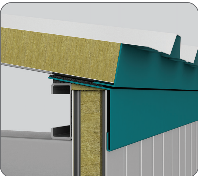
Ön Alın Kaplama Detayı / Front Covering Detail
