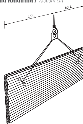
Şekil 9 D - Vakumlu Kaldırma / Vacuum Lift
