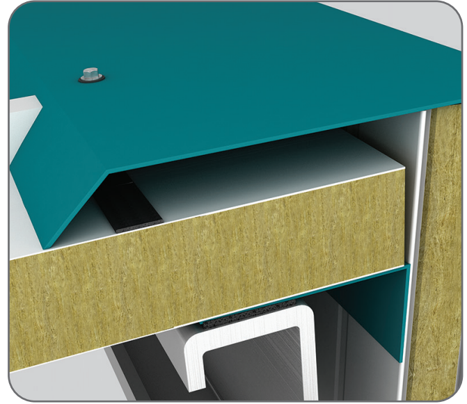
Yarım Mahya Detayı / Semi Ridge Detail
