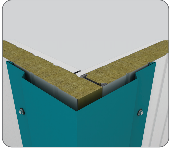
Dış Köşe Detayı / Outer Corner Detail
