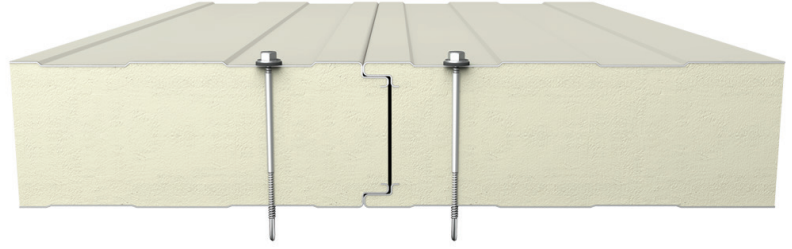
Birleşim Detayı / Connection Detail
