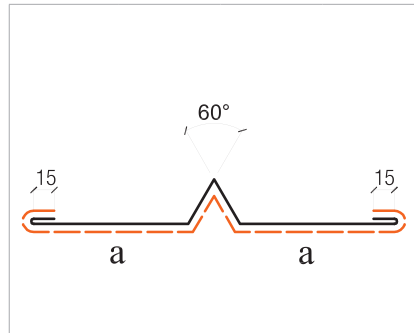
Dilatasyon Derz Profili / Dilatasyon Expansion Profile
