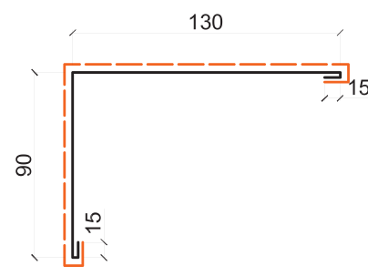
Soğuk Oda Depo Dış Köşe Profili Cold Storage Outer Corner Profile
