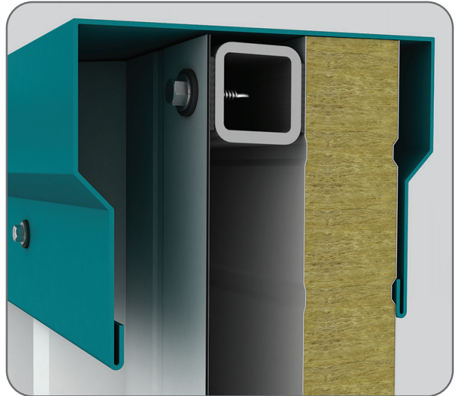
Harpuşta Detayı / Protection Cap Detail
