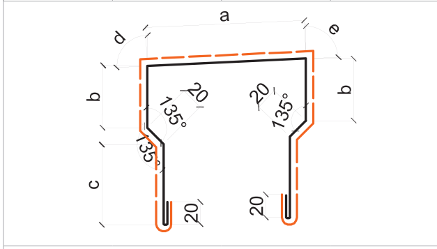
Harpuşta Profili / Eaves Gutter Parapet Profile
