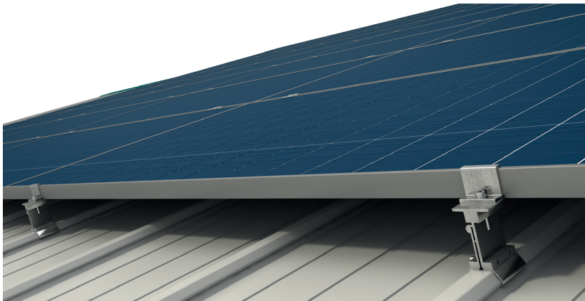
Profilsiz Bağlantı Aparatı / Connection Apparatus without Profile
