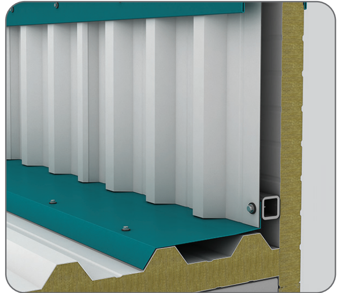
Kalkan Duvar Çatı Birleşimi-2 / Shield Roof-Wall Connection Detail-2
