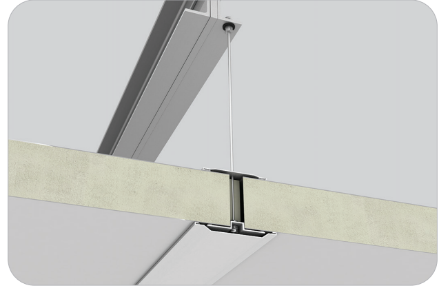
Soğuk Oda Askı Tiji Detayı-2 / Cold Room Suspender Tiji Detail-2
