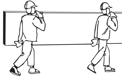
Şekil 9 B - Panel Taşıma / Manuel Transfer
