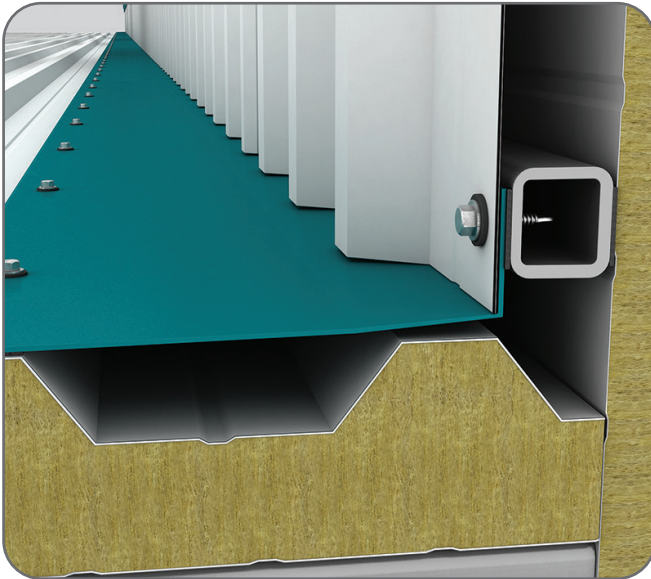
Kalkan Duvar Çatı Birleşimi-1 / Shield Roof-Wall Connection Detail-1
